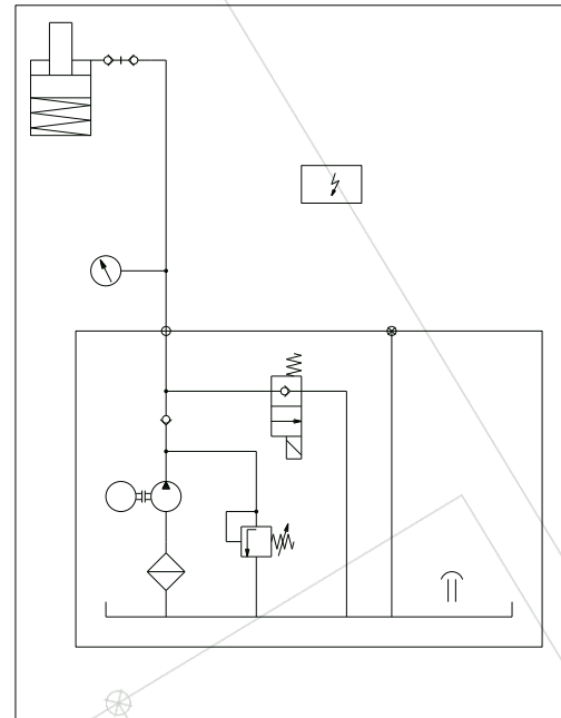
Hydraulisches Schema
